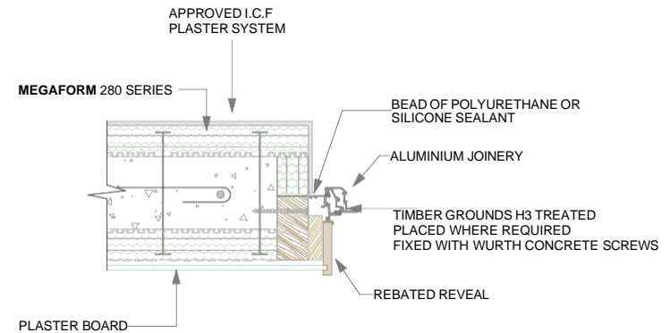
WINDOW JAMB
