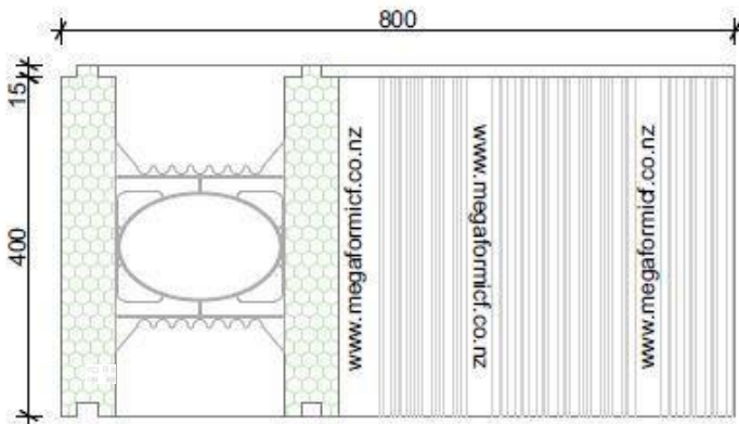
ELEVATION B
