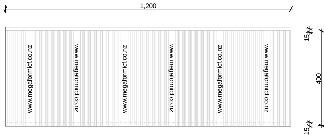
ELEVATION
