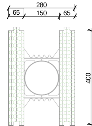
END ELEVATION
